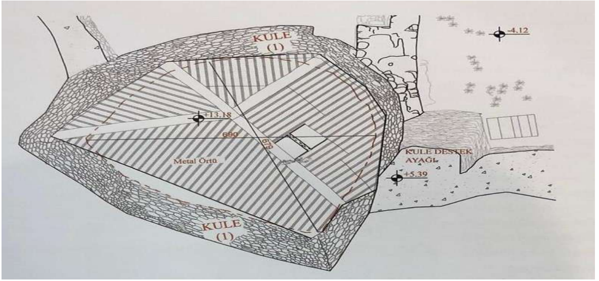
Resim 2: 1 No.lu Kule Planı
